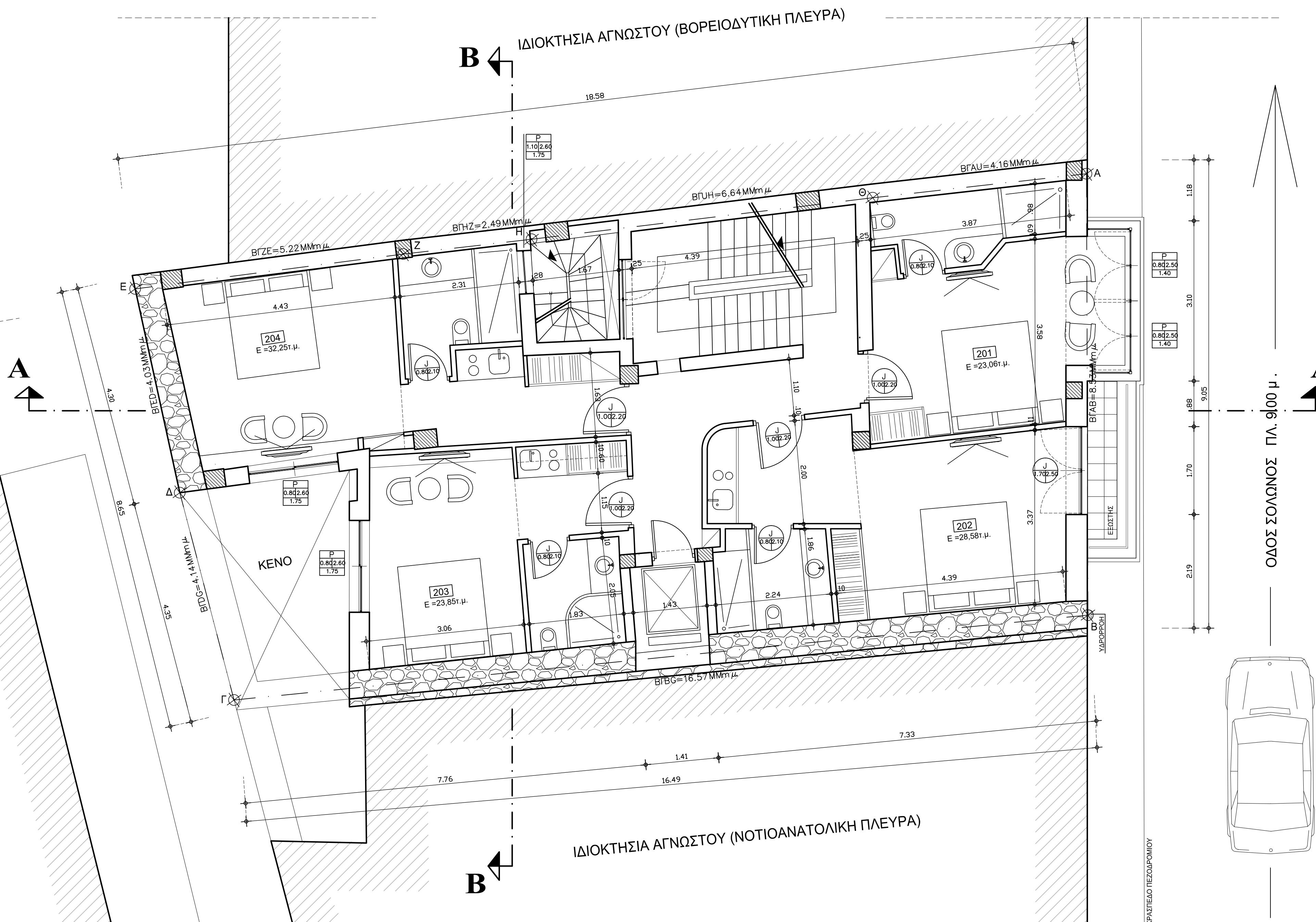
ΚΑΤΟΨΗ Β' ΟΡΟΦΟΥ
